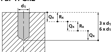
Spanbruchzyklus
