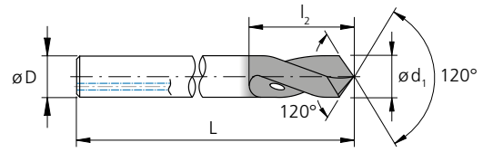
Ausführung: d_1 = 3.0 bis 10.0 mm
