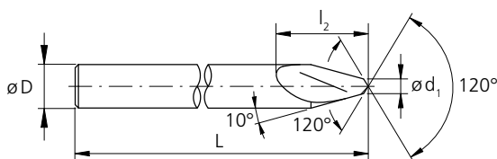
Ausführung: d_1 = 0.5 und 1.0 mm
