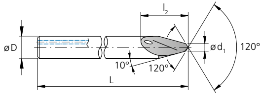
Ausführung: d_1 = 0.5 bis 2.0 mm
